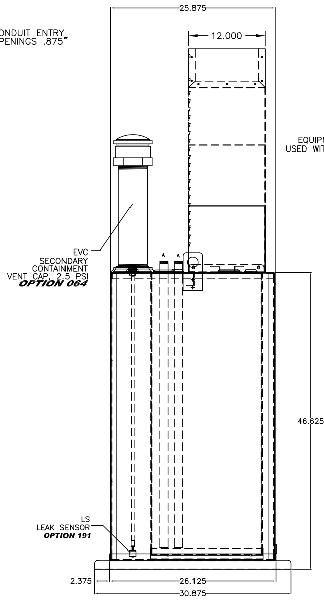
L.H. VIEW
