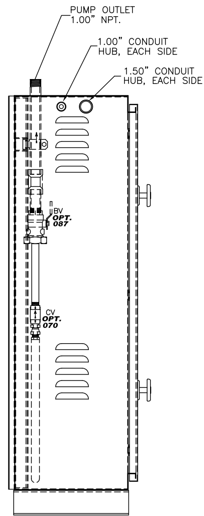
LEFT SIDE
